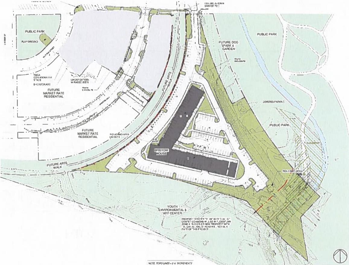
Figure 2. Bristow Commons Site Plan
