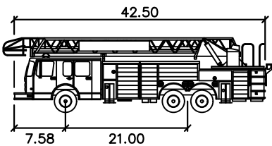
CSFD Apparatus
